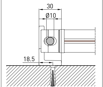
supporto a nicchia - niche bracket B-B
